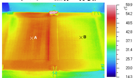
サーモビューアによる撮影画像 (レフランプ照射10分後)
